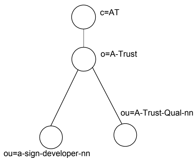
Abbildung 2 a.trust Verzeichnisbaum
